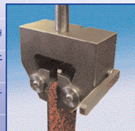
Tensile testing
